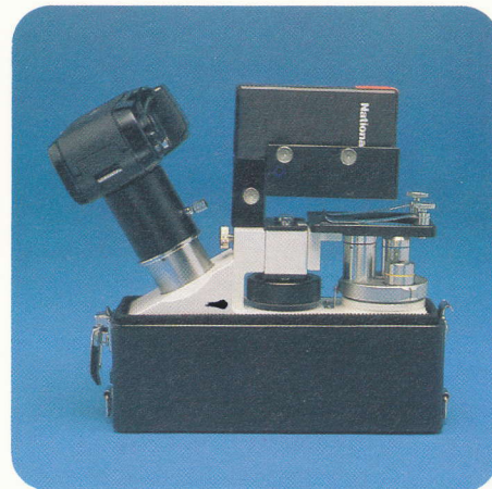
Exkursions-Mikroskop mit Pentax Auto 110, Kamera-Adapter, Batterie-Leuchte.
